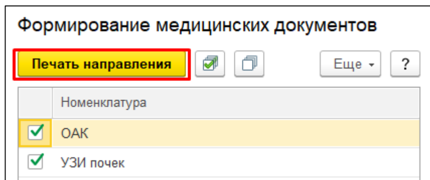
Рисунок 17 – Печать направления
