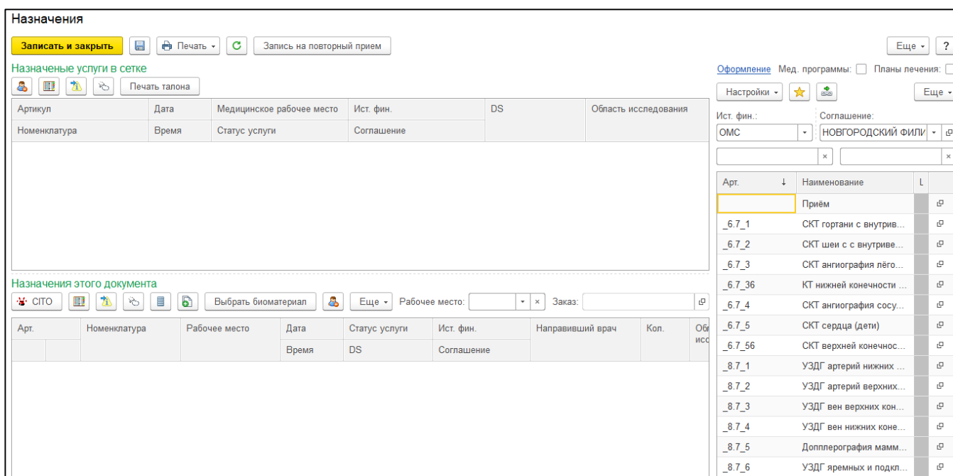
Рисунок 4 – Форма «Назначения»
