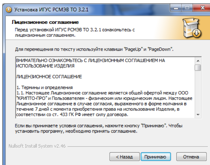
Рисунок 4.3. – Лицензионное соглашение
