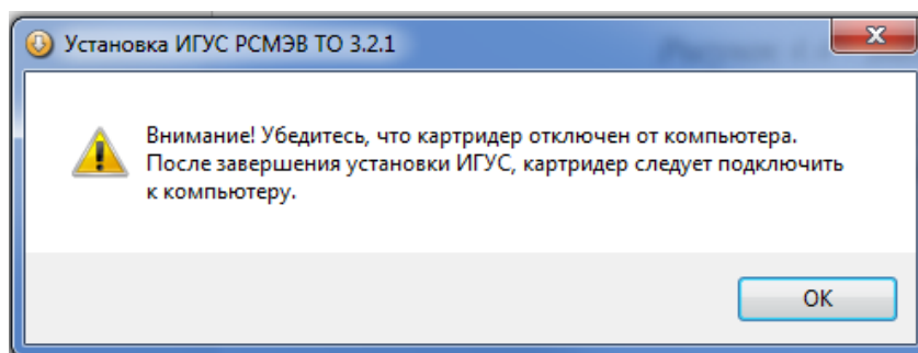
Рисунок 4.5 – Информационное окно
